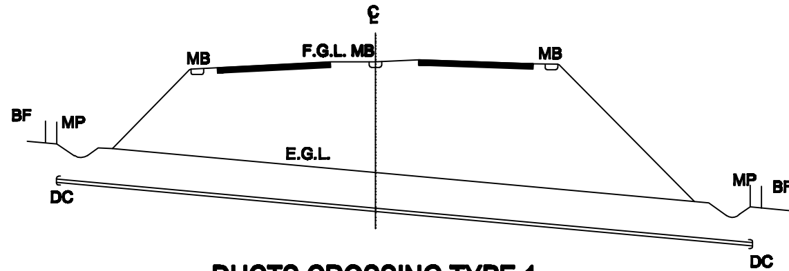
DUCTS CROSSING TYPE 1. (FILL AREAS) N.T.S.
