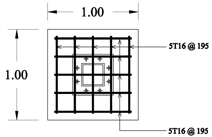
Plan A-A
